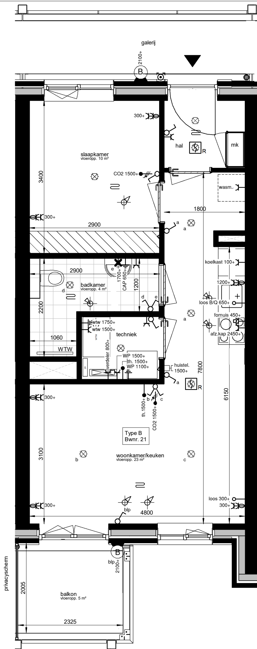
derde verdieping
