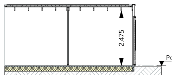
Doorsnede B-B schaal 1:100
