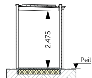
Doorsnede A-A schaal 1:100
