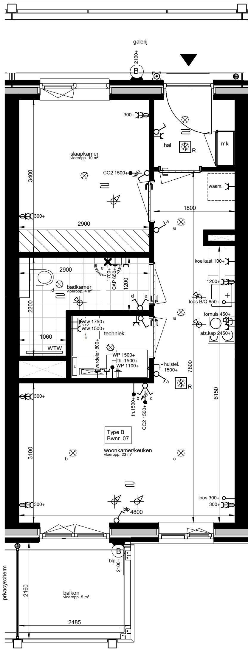
eerste verdieping
