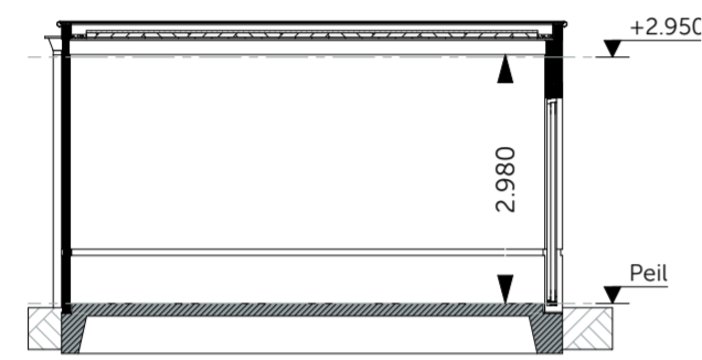
Doorsnede A-A schaal 1:100
