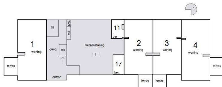
begane grond
